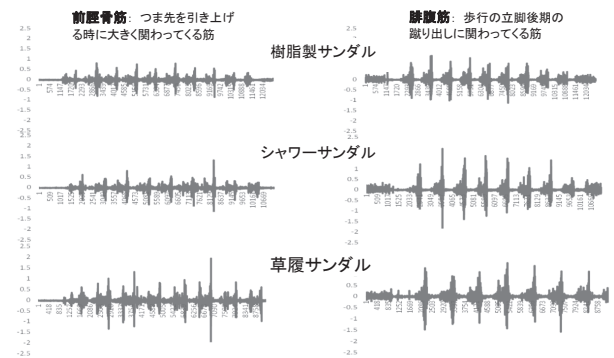
図10 履物による歩行時筋活動の相違
